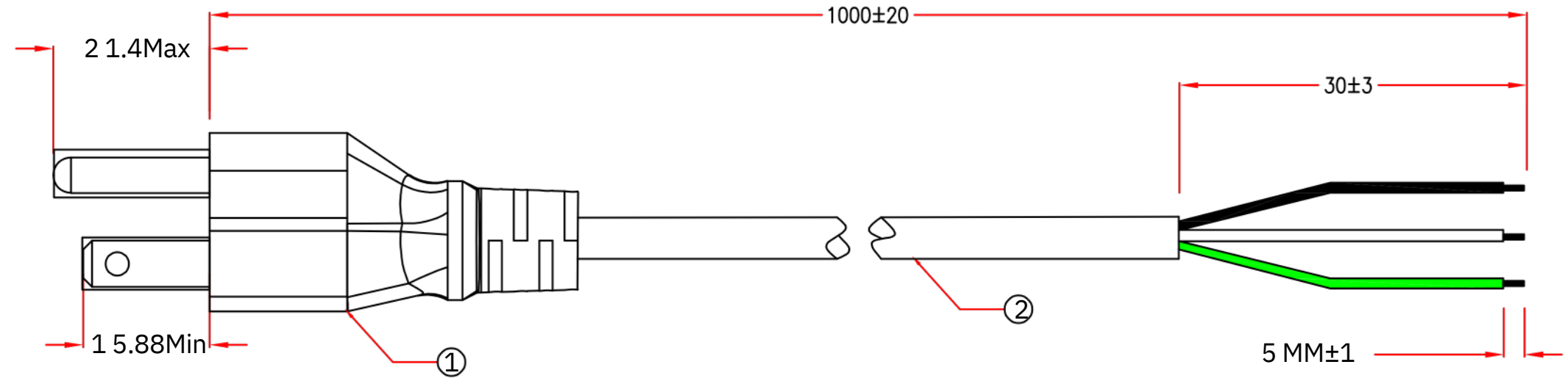
P1:UL 3Pin
