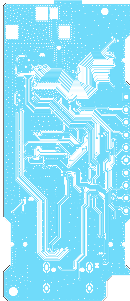
Layer 2 (Scale 2.5:1)
