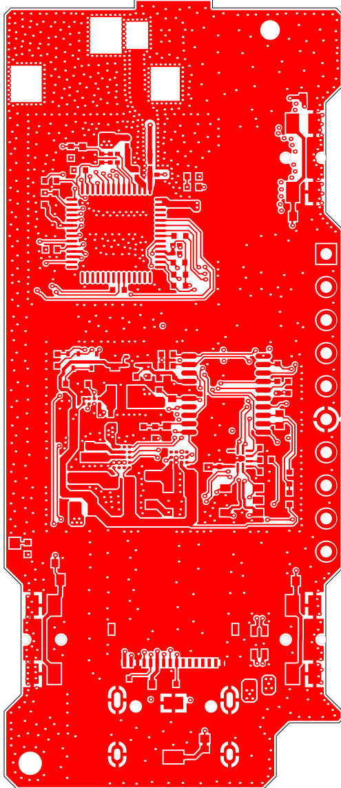
Top/Sig1 (Scale 2.5:1)
